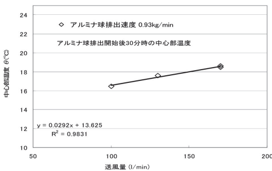
図14 中心部温度に及ぼす送風量の影響
