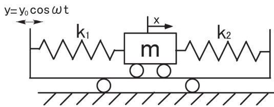
図 2 振動系モデル
