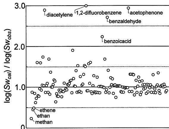
図 5 溶解度の推算値と文献値の誤差ならびに相関精度の悪い有機化合物
