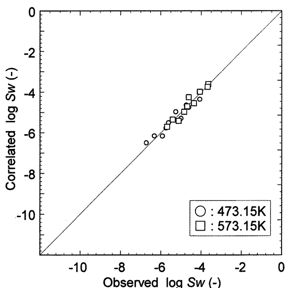
図 6 パラメーターセット A' : [TMS- E_{dc} -CN-Temp] を用いて推算した高温水への溶解度と文献値
