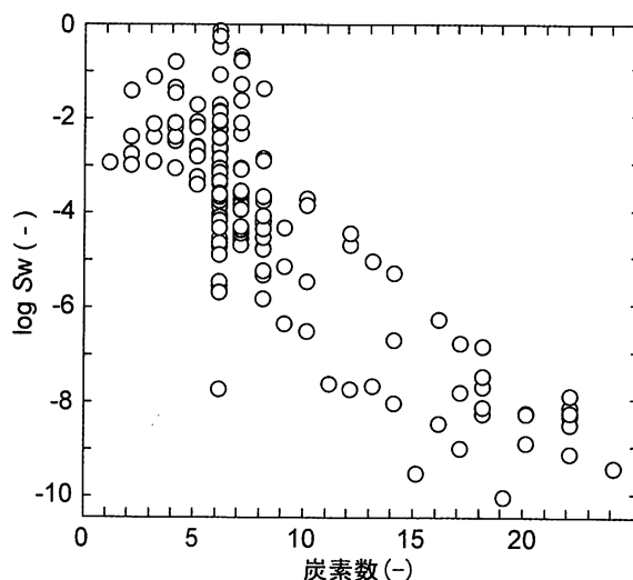
図2 炭素数の溶解度への寄与割合
