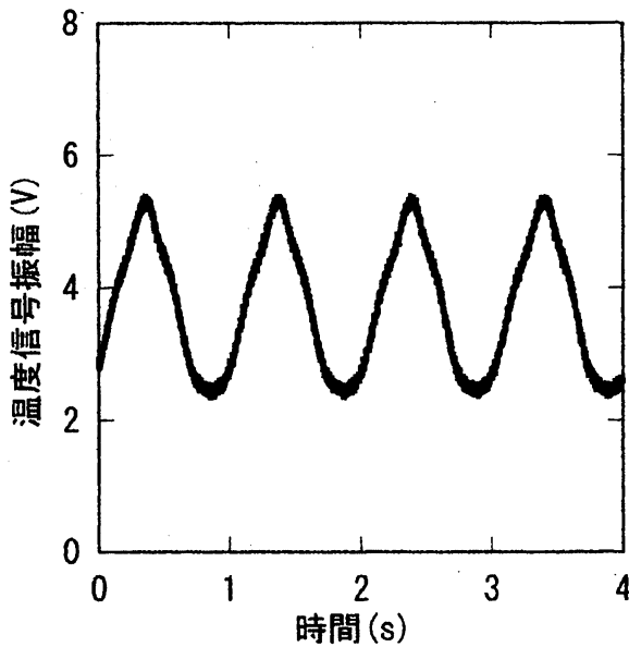
図7 温度計からの出力波形 (1000mHz)
