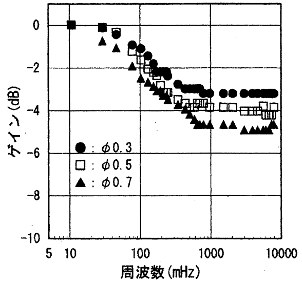
図8 プロブ直径の違いによる低周波の特性の変化
