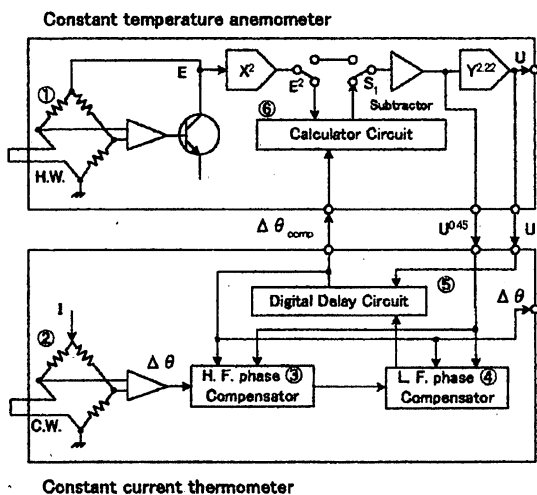
図1 二線式温度流速計ブロックダイアグラム
