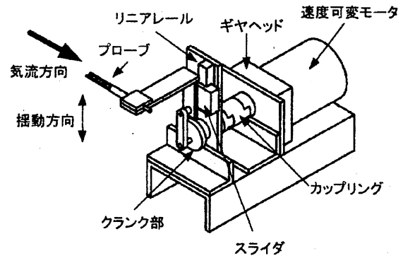
図4 新しい検定装置
