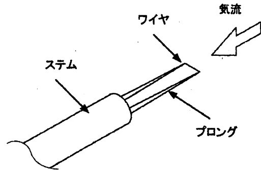
図2 使用した温度プローブ
