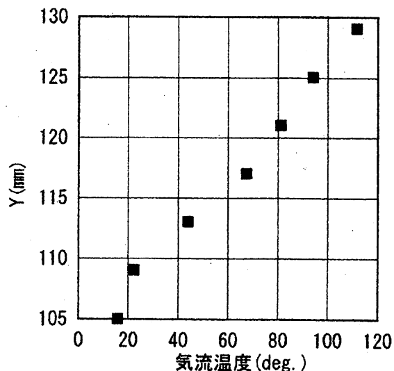
図5 風洞出平均温度分
