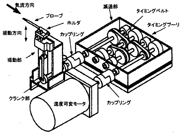
図3 従来の検定装置
